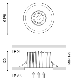
DUOM0 IP65 / IP20
