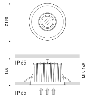
DUOM0 IP65 / IP65
